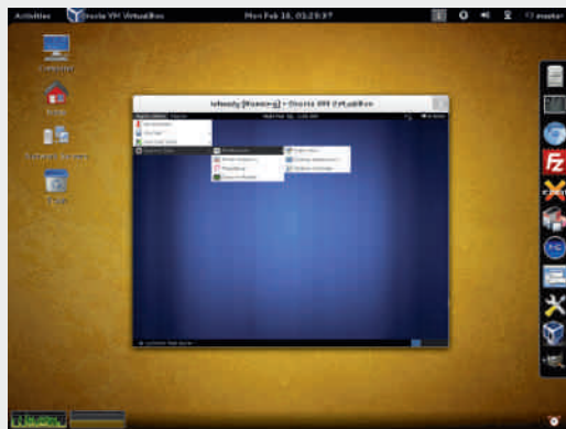
Slika 3
