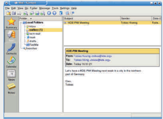
Slika 4: Kmail
