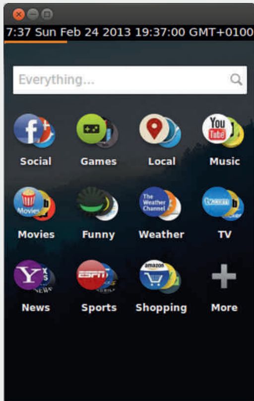
Slika 2: Pretraga
