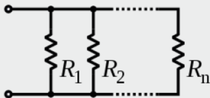
Slika 5: paralelna veza otpornika
