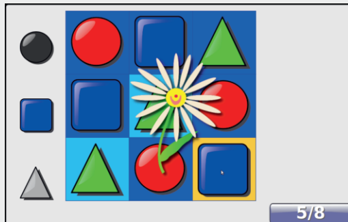
Slika 10 GCompris Sudoku
