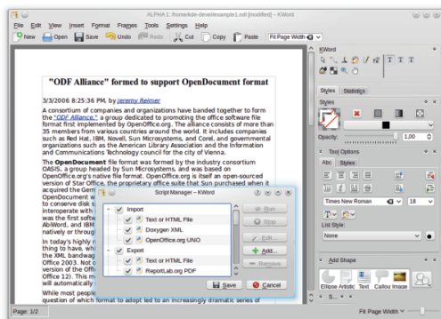
Slika 17: KOffice
