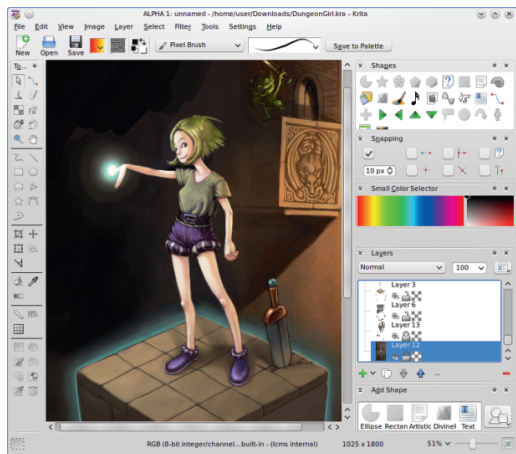
Slika 13: Krita
