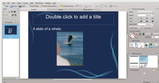
Slika 9: Stage
