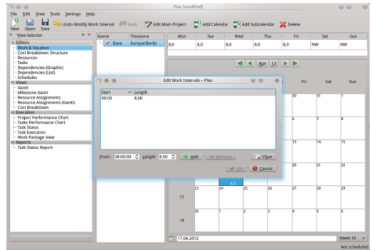
Slika 10: Plan
