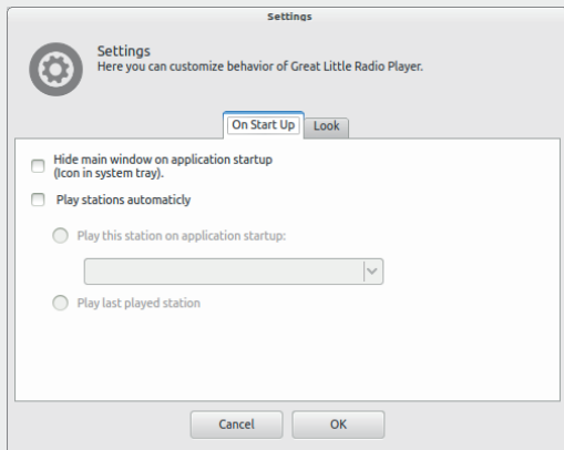
Slika 3: Sekcija podešavanja
