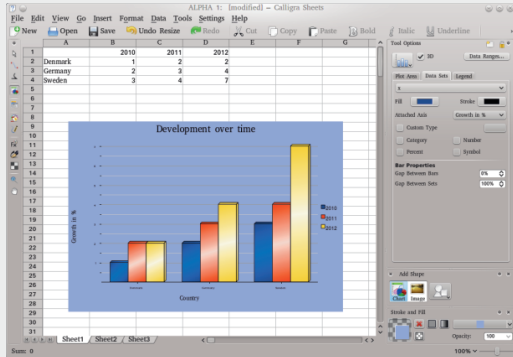
Slika 8: Sheets
