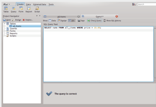
Slika 14: Kexi
