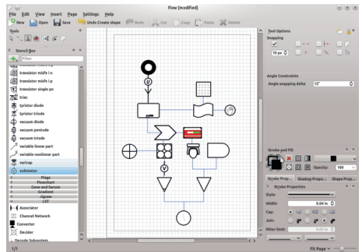
Slika 11: Flow
