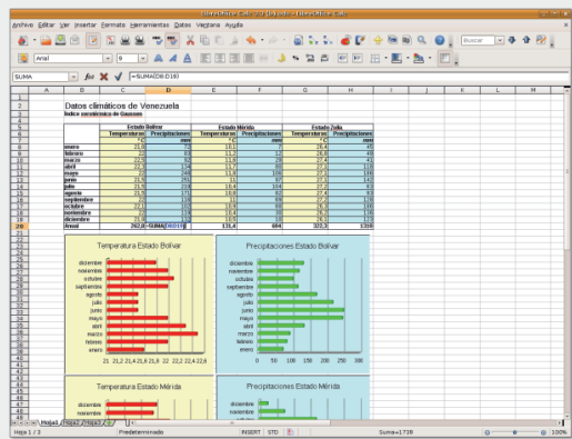
Slika 2: Calc
