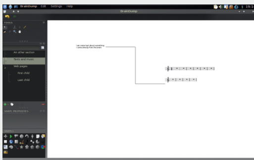
Slika 15: Braindump
