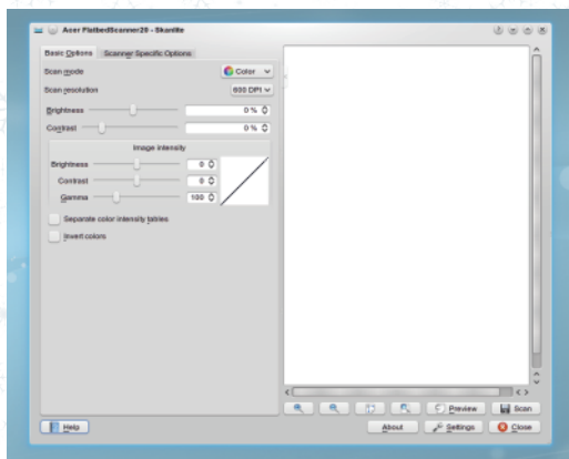
Slika 8: Scanlite
