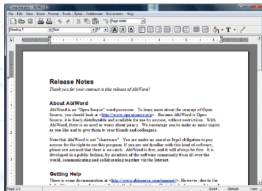
Слика 2: AbiWord
