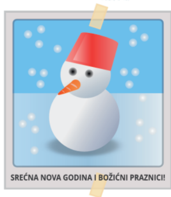
Слика 8: Честитка!
