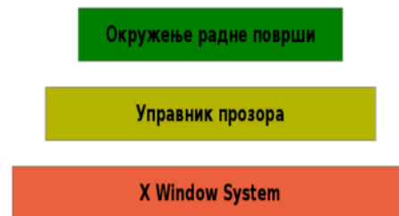
Слика 1. Хијерархија графичког корисничког интерфејса
